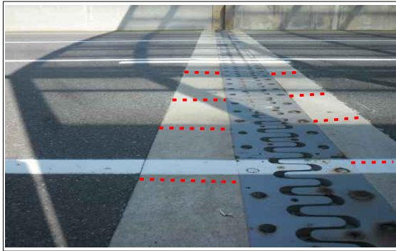
하행선 A2 신축이음 후타재 균열 (폭0.2mm)
