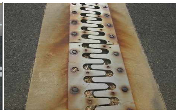
상행선 A1 신축이음 본체 고정볼트 녹발생
