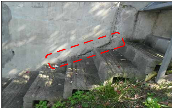
하행선 A1 우측 날개벽 날개벽과 점검계단 이격
