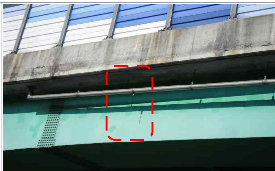
하행선 S2 배수관 연결재 탈락
