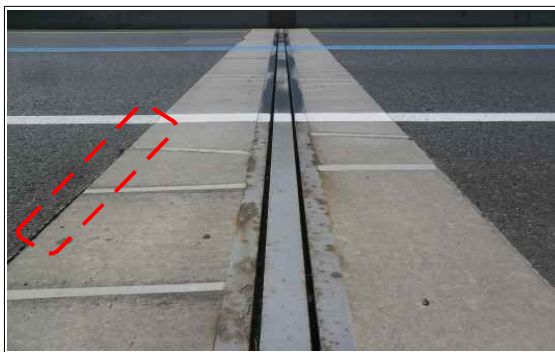
상행선 A1 신축이음 후타재 접속부 이격
