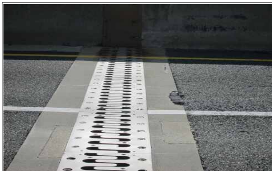
상행선 A1 신축이음 후타재 파손
